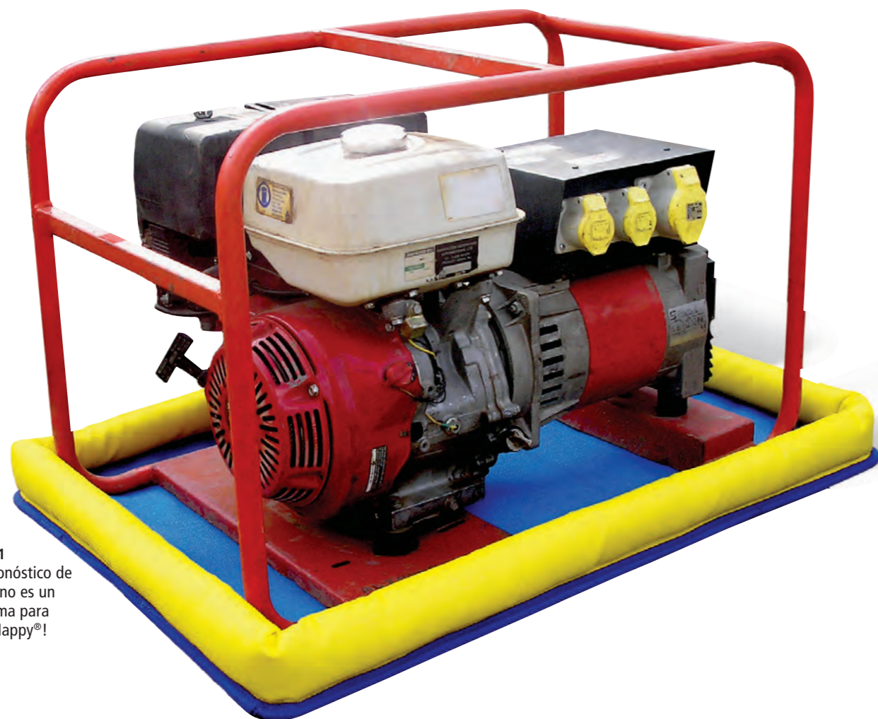
RFLE700 Se pueden añadir revestimiento Plant Nappy® (se venden por separado) para ampliar la vida útil.
